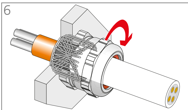
Druckschraube mit dem empfohlenen Anzugsdrehmoment anziehen
