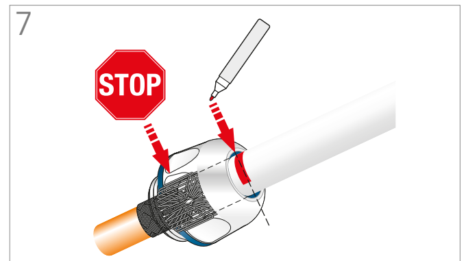
Markieren, wenn der Kabelmantel die Feder berührt
