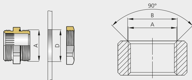
Abb. 1 – Durchgangsbohrung Fig. 1 – Through-hole
