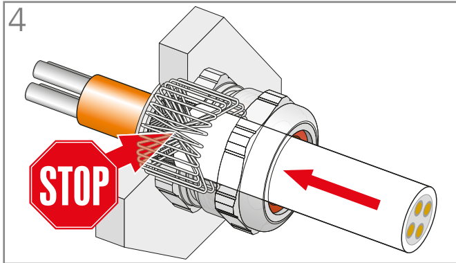
Kabel weiter einführen, bis der Kabelmantel die Feder berührt Continue inserting the cable until the sheathing touches the spring
