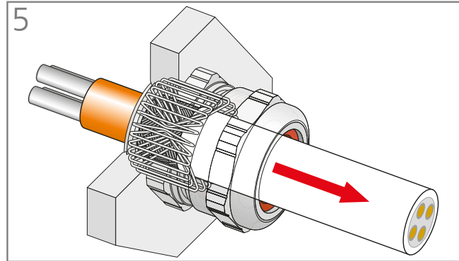
Kabel um ca. 2 mm zurückziehen, sodass die Feder keinen Kontakt zum Kabelmantel hat Pull the cable back approx. 2 mm so that the spring does not touch the cable shield
